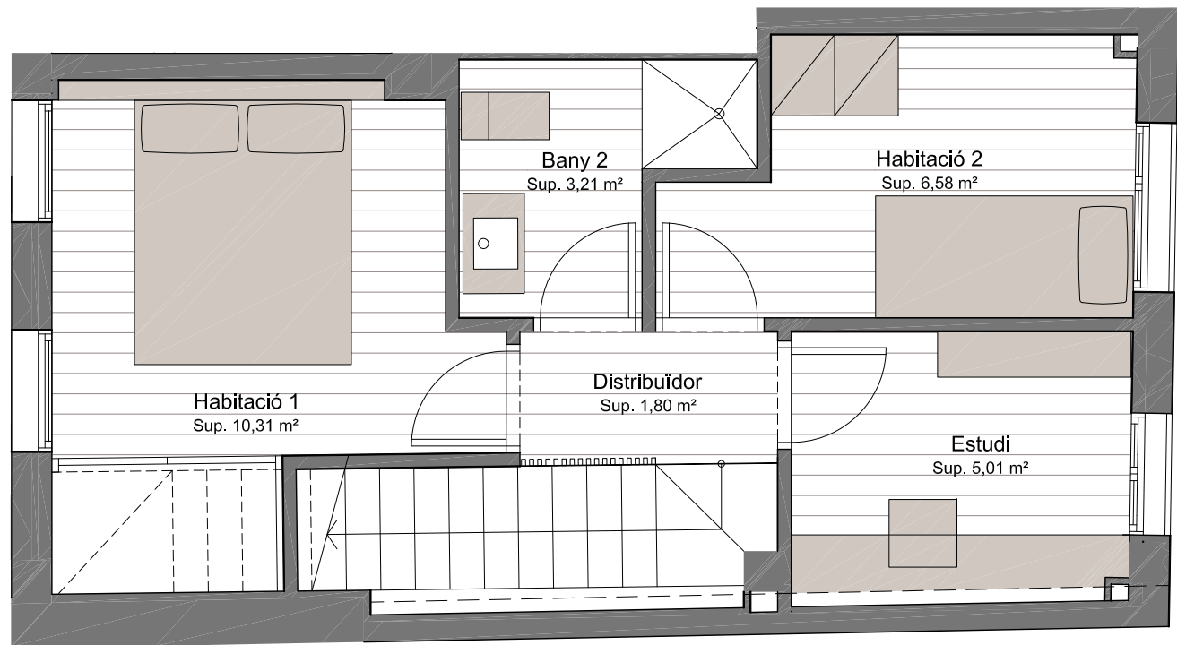
PLANTA BAIXA
