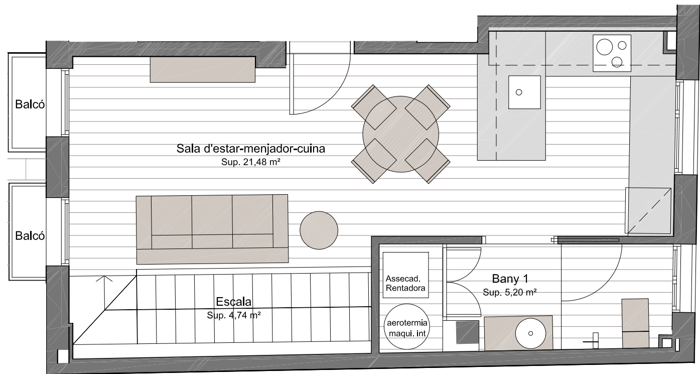
PLANTA 1ª
